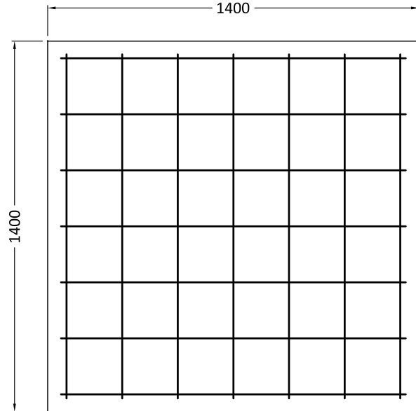
SNIÐ B 1:20
