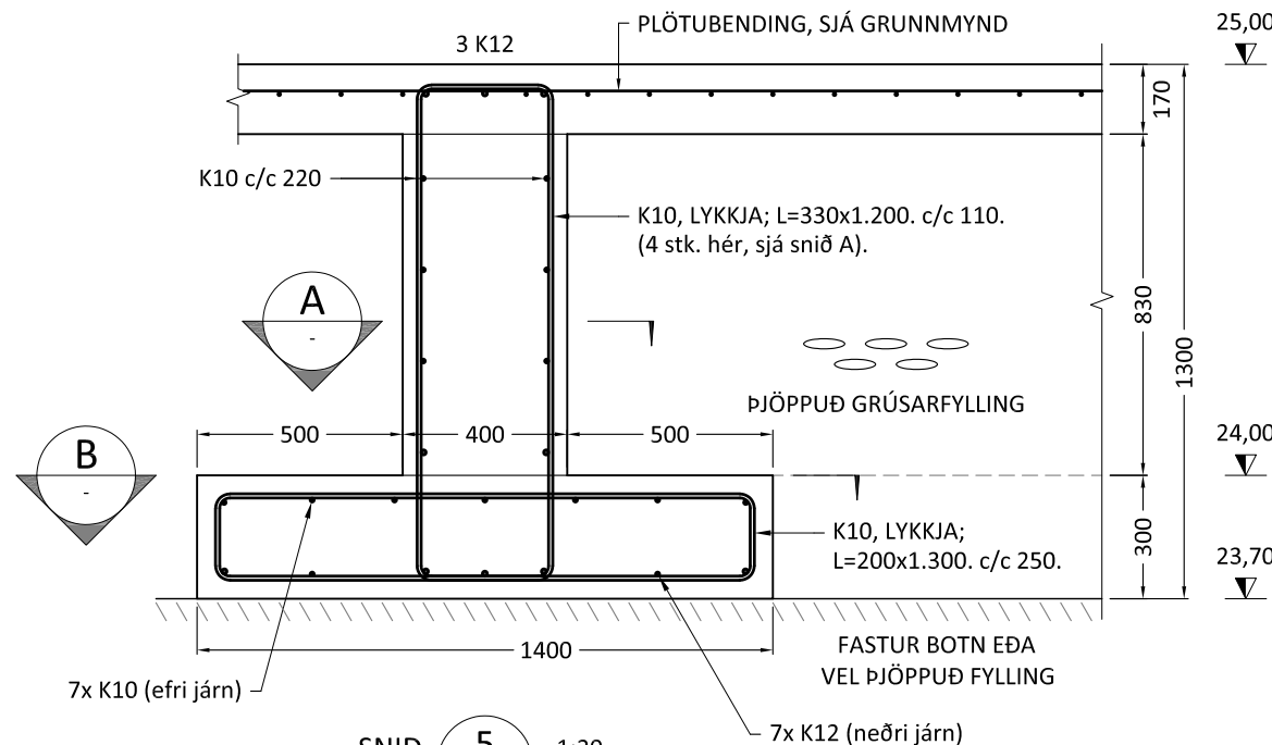
SNIÐ 5 1:20 120-01
