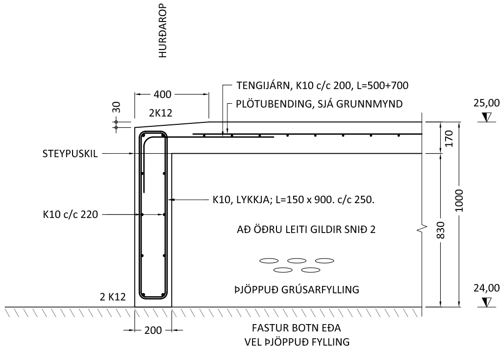
SNIÐ 2b 1:20 120-01a 120-01b
