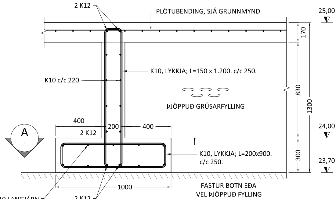
SNIÐ 4a 1:20 120-01
