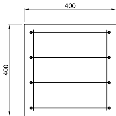
SNIÐ A 1:10
