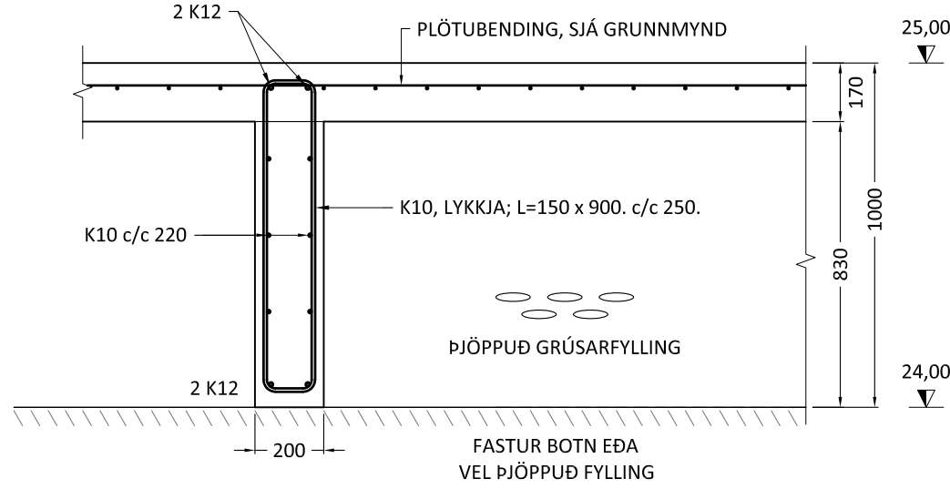
SNIÐ 4 1:20 120-01
