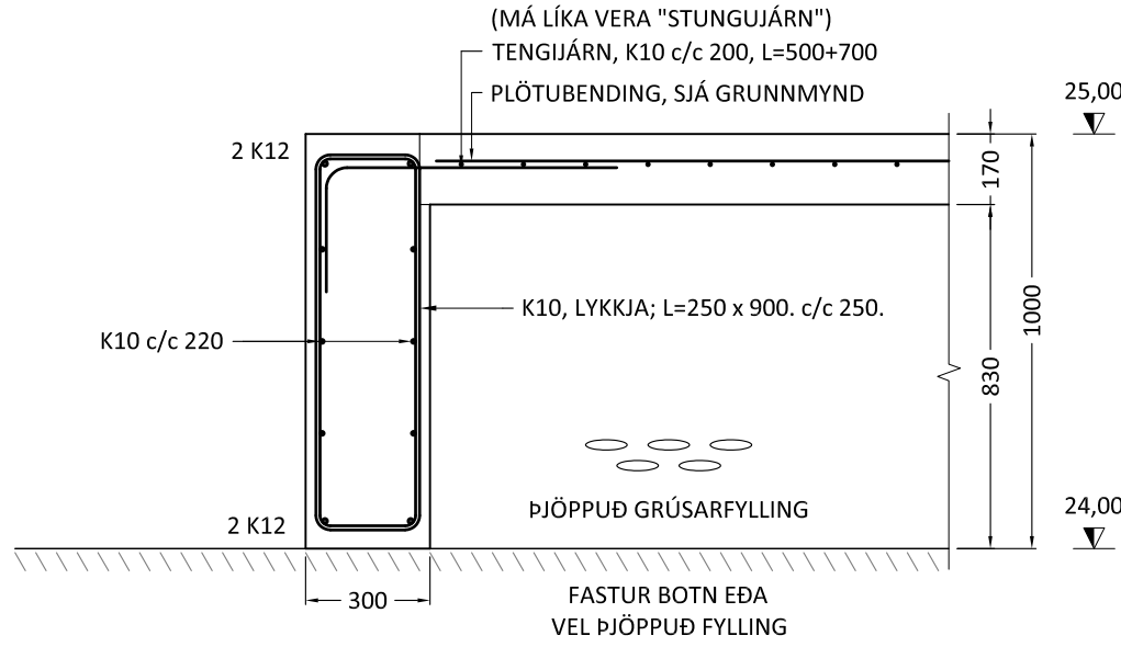
SNIÐ 3 1:20 120-01a 120-01b
